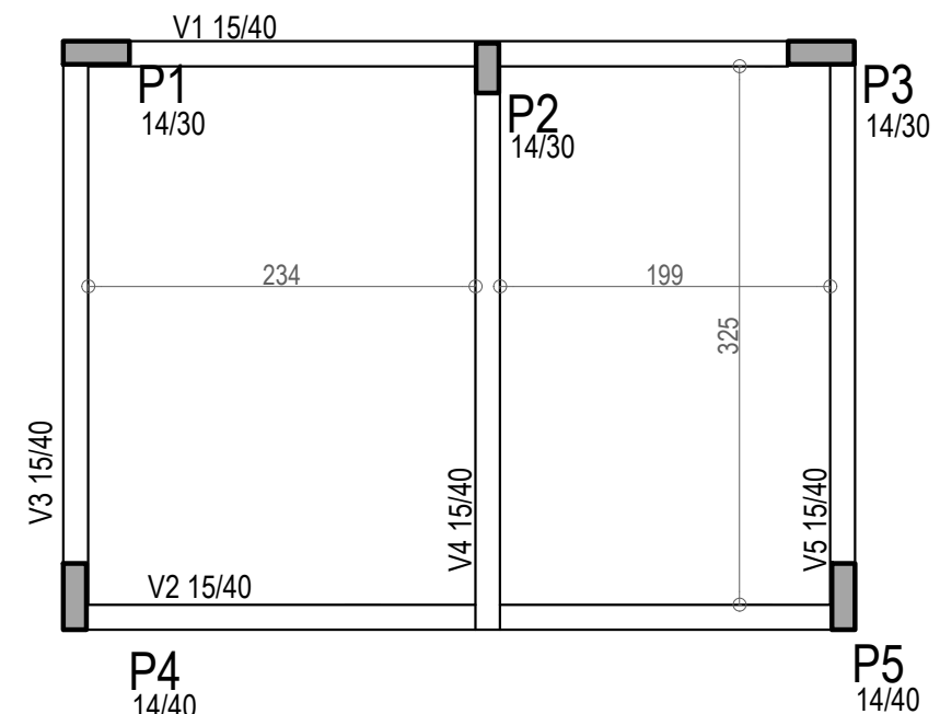
PLANTA DE FORMA COBERTURA ESC:1/50
