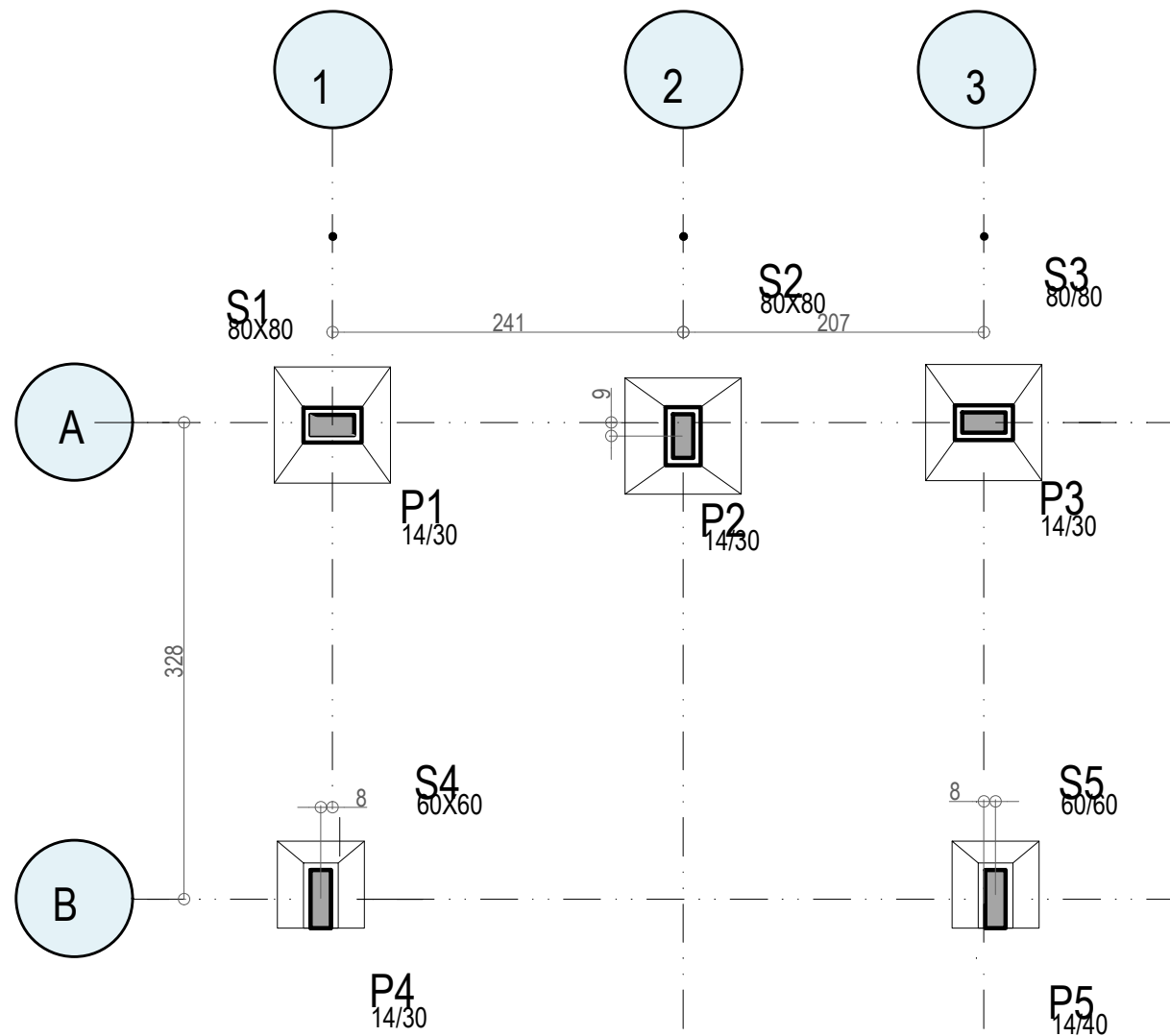
PLANTA DE LOCAÇÃO ESC:1/50
