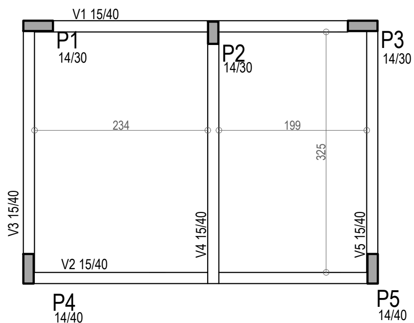
PLANTA DE FORMA TÉRREO ESC:1/50
