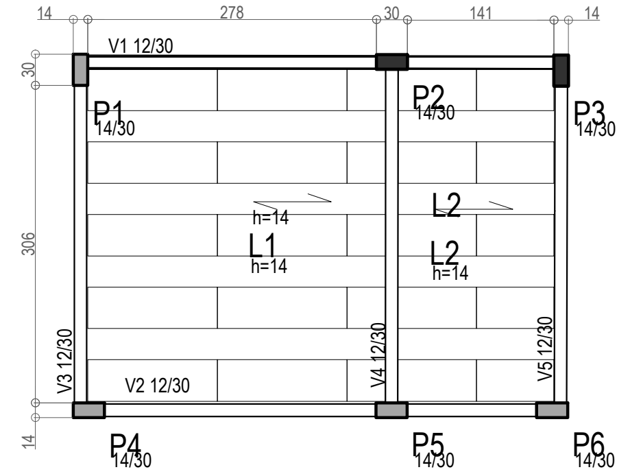
PLANTA DE FORMA COBERTURA ESC:1/50
