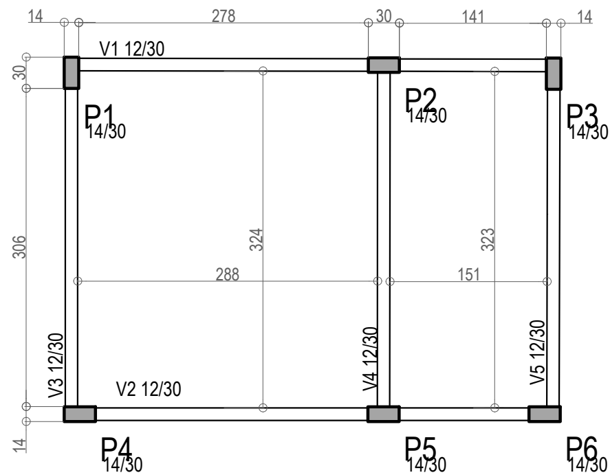
PLANTA DE LOCAÇÃO ESC:1/50
