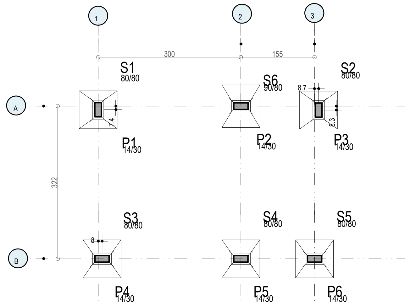
PLANTA DE LOCAÇÃO ESC:1/50
