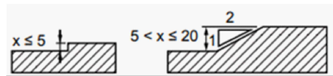
Detalhe do chanfro Sem escala
