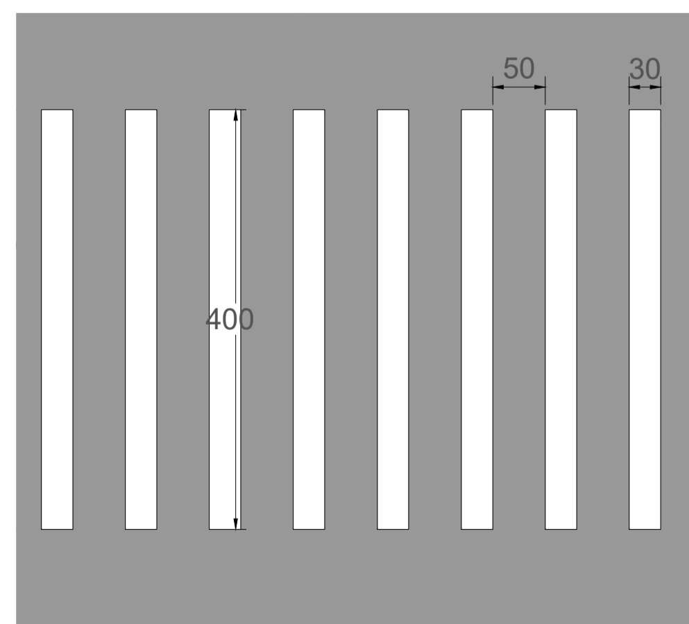
Detalhe da faixa de travessia de pedestres Esc:1/50
