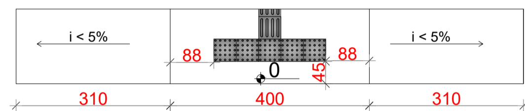
Detalhe da calçada Esc:1/75
