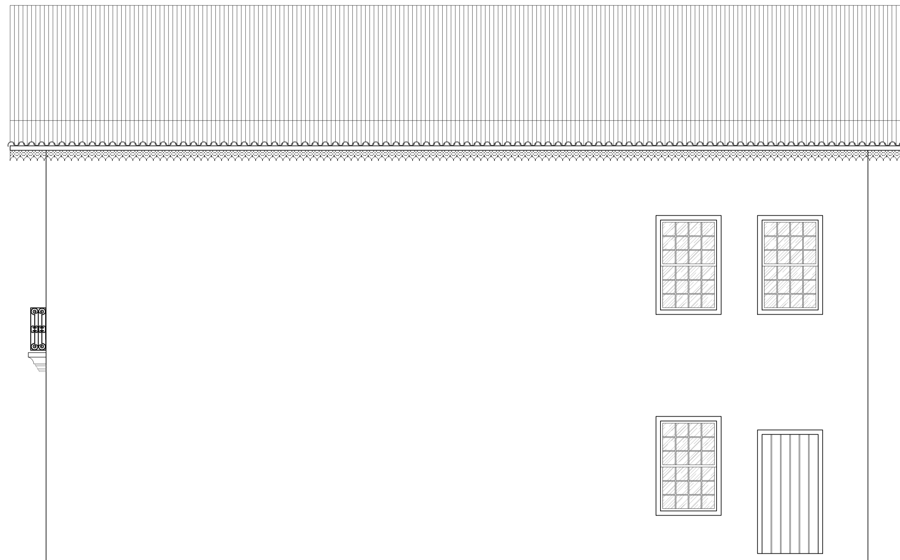
FACHADA LATERAL ESQUERDA ESCALA: 1/50
