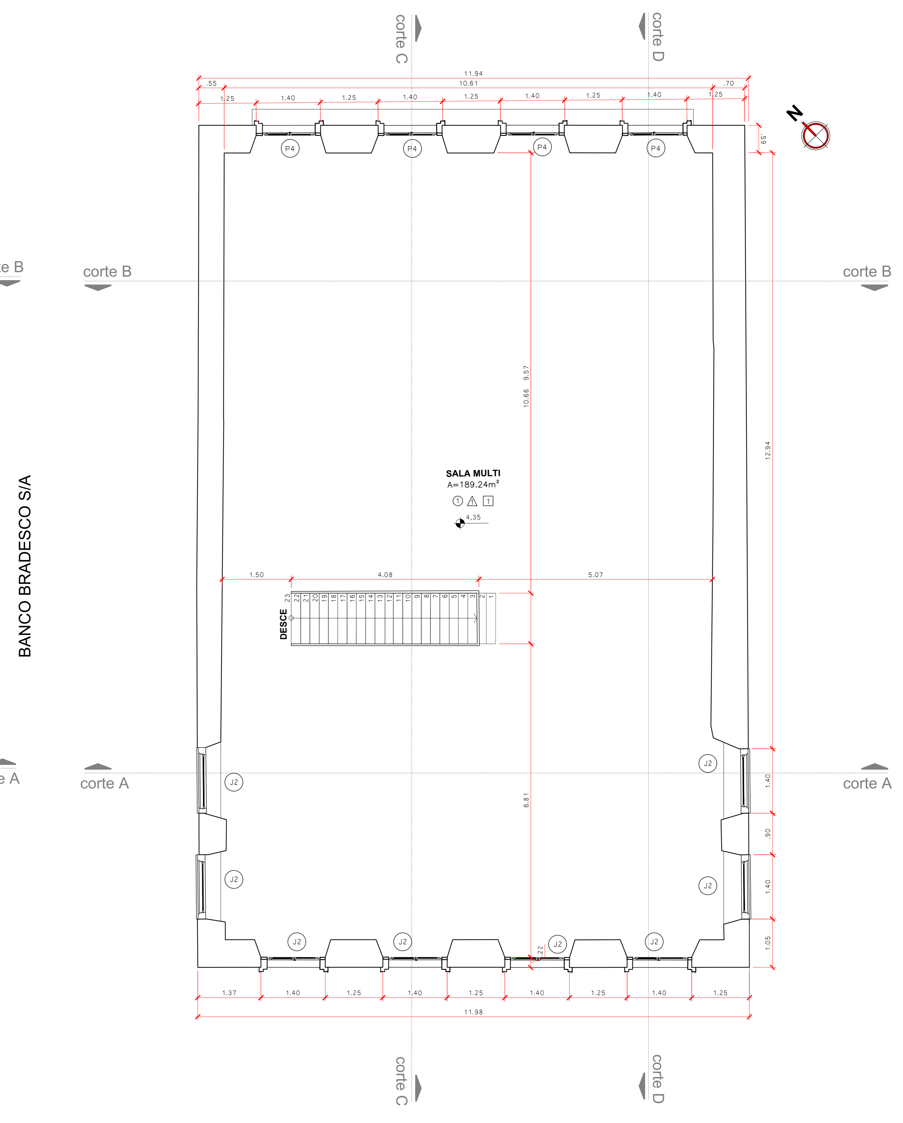
PLANTA BAIXA PAVTO. SUPERIOR ESCALA: 1/50
