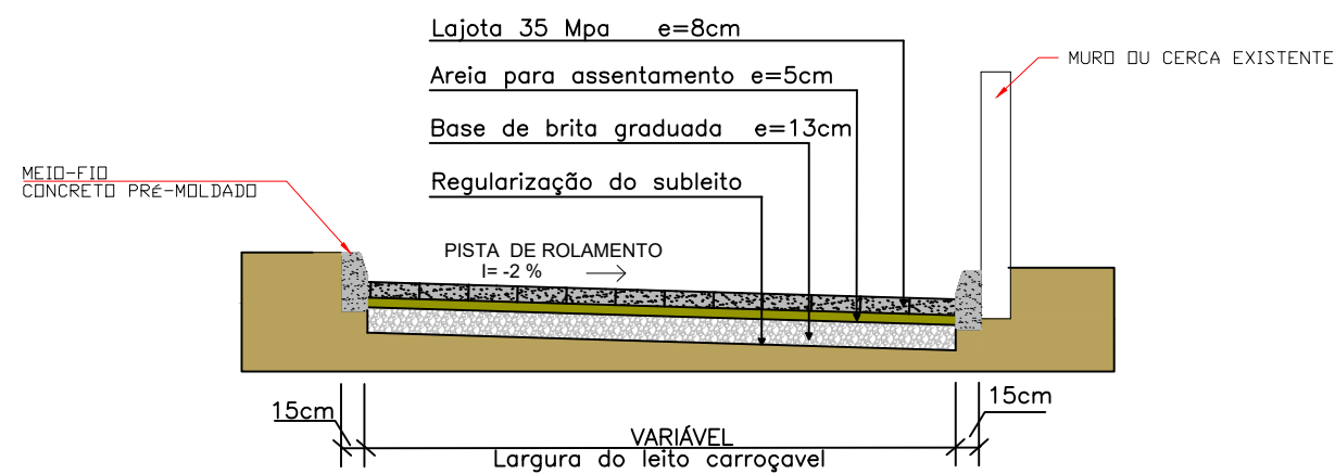
DETALHE 1 - SEÇÃO TIPO DO PAVIMENTO SEM ESCALA
