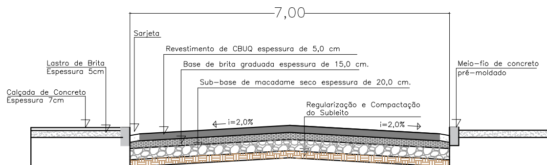
SEÇÃO TIPO DO PAVIMENTO SEM ESCALA
