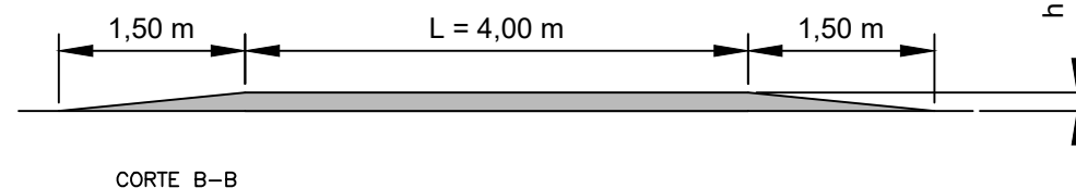
CORTE B-B
