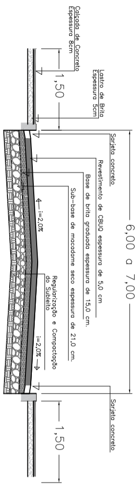
DETALHE 01 - SEÇÃO TIPO DA VIA TRECHO 2 - PP a 11+09 SEÇÃO TIPO DO PAVIMENTO SEM ESCALA
